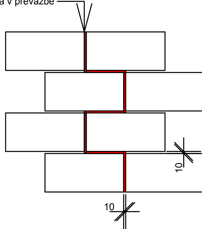
Dilatační spára v převazbě
