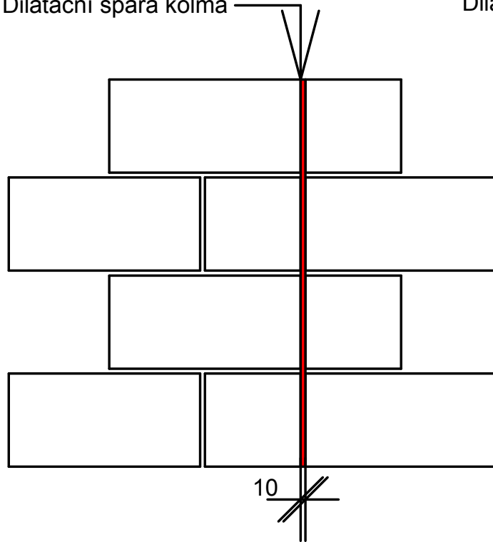
Dilatační spára kolmá
